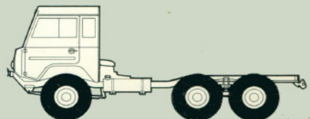
C306 6x6 Fahrgestell mit Fahrerhaus.
