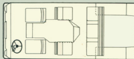
C303 4x4 mit offenem Aufbau
